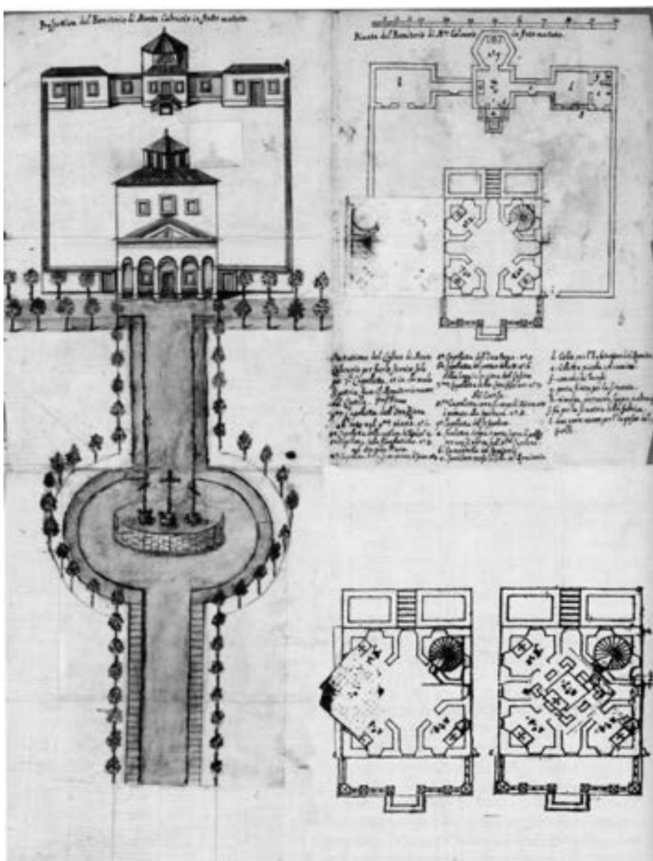
Fig. 11. Santo Deserto di Monteverginio, Progetto di ampliamento del romitorio del Monte Calvario e della cordonata di accesso: vista a volo d'uccello, piante del piano terreno, del primo e secondo piano, penna e acquerello, fine sec. XVII (Roma, Archivio di Stato, Carmelitani Scalzi, S. Maria della Vittoria, fasc. 524, n. 10).
