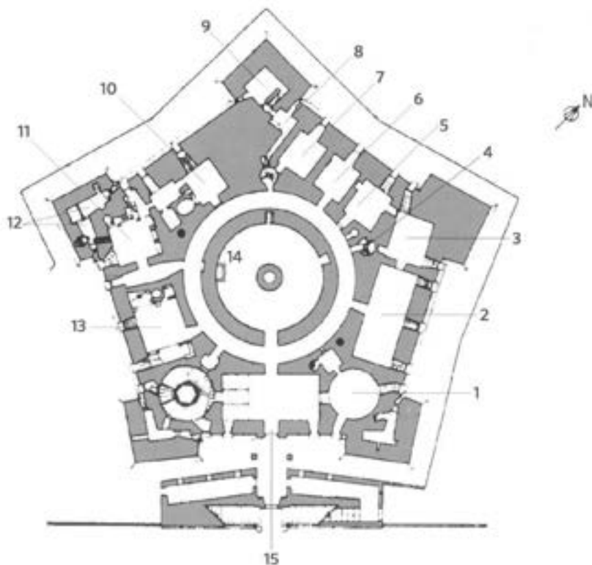
Fig. 12. Cantine del palazzo Farnese a Caprarola con indicazione delle funzioni nei luoghi principali: 1-Dispensa; 2-Tinello per la famiglia; 3-Stanza 'dei piatti di stagno'; 4-Pozzo; 5-Stanza del mulino; 6-Stanza dell'olio; 7-Stanza 'delli piatti'; 8-Stufa del Cardinale; 9-Conserva; 10-Stanza del forno; 11-Cucina del Cardinale; 12-'Pasticceria'; 13-Cucina per la famiglia; 14-Abbeveratoio; 15-Portale 'del Facchino'.
