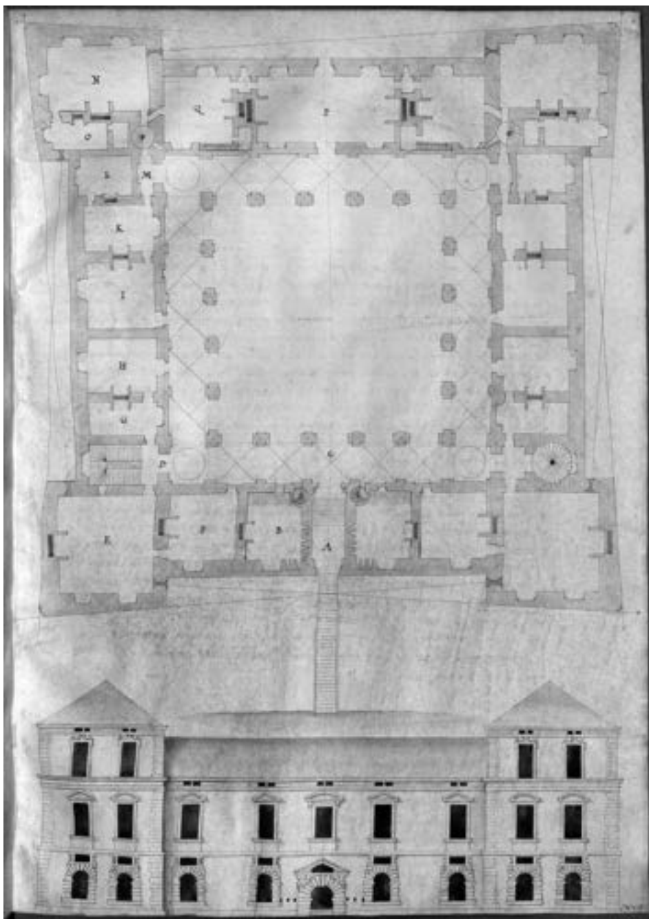
Fig. 3. Sebastiano Serlio, Della casa del principe illustre in modo di fortezza , in Sesto libro d'architettura. Delle habitationi fuori e dentro delle città , ms. Bayerische StaatsBibliothek, Hss Cod. Icon 189, tav. XVIII.
