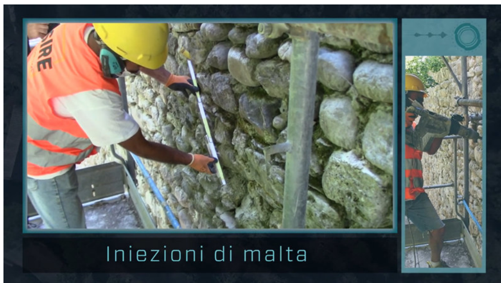
3: Operazioni volte alla realizzazione dei fori nella muratura per la successiva iniezione di malta fluida, tratte dalla Puntata 8 - I consolidamenti della cerchia muraria .
