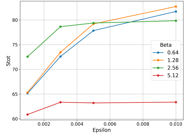
(d) S_{tot} , Entropic Student.
