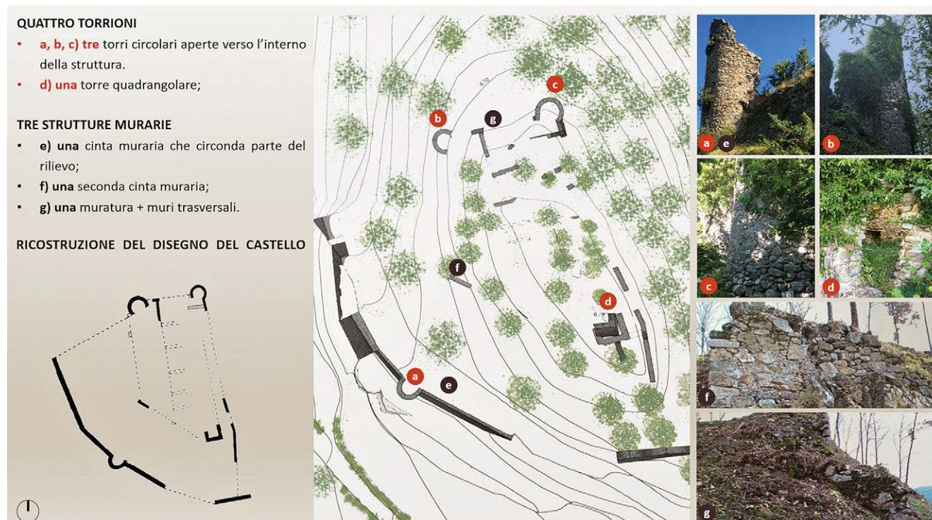
fig. 17 – Una delle tante schede tecniche riguardanti i castelli e i complessi fortificati indagati durante la campagna del 2017. In particolare sono evidenziate le torri, le strutture murarie superstiti e la sezione orizzontale del castello di Perlo (elaborazione grafica degli/delle specializzandi/e).
