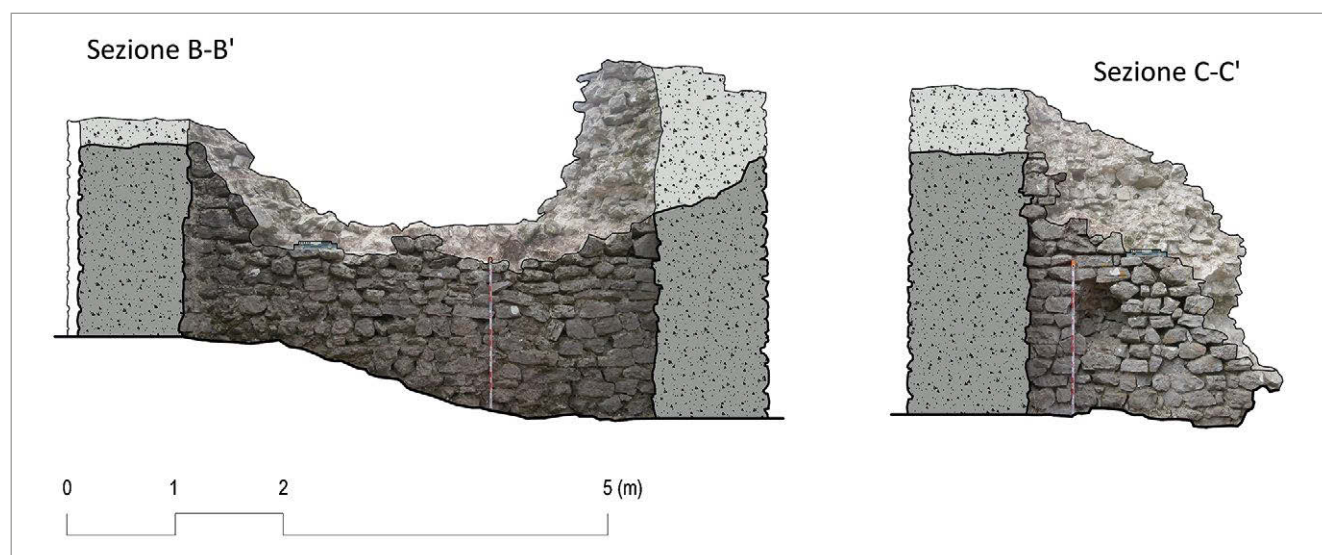
fig. 6 – Rilievo della torre sud della cinta, la quale è stata sottoposta a una pulitura archeologica e delle creste murarie durante gli anni di attività della Scuola di Specializzazione in Beni Architettonici e del Paesaggio del Politecnico di Torino.
