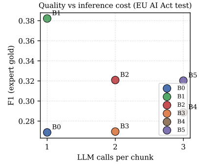
Fig. 3. F1 vs. LLM calls per chunk (B0–B5 ablation).
