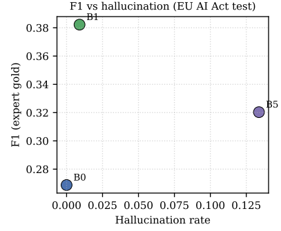
Fig. 4. F1 vs. hallucination rate trade-off (EU AI Act test).
