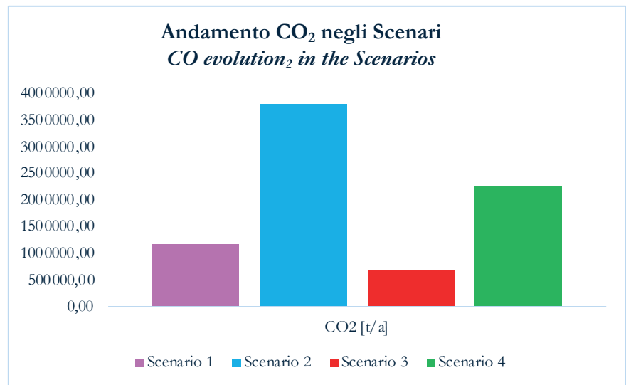
Figura 13 - Andamento CO 2 nei due scenari a livello regionale. Figure 13 - CO 2 trends in the two scenarios at regional level.
