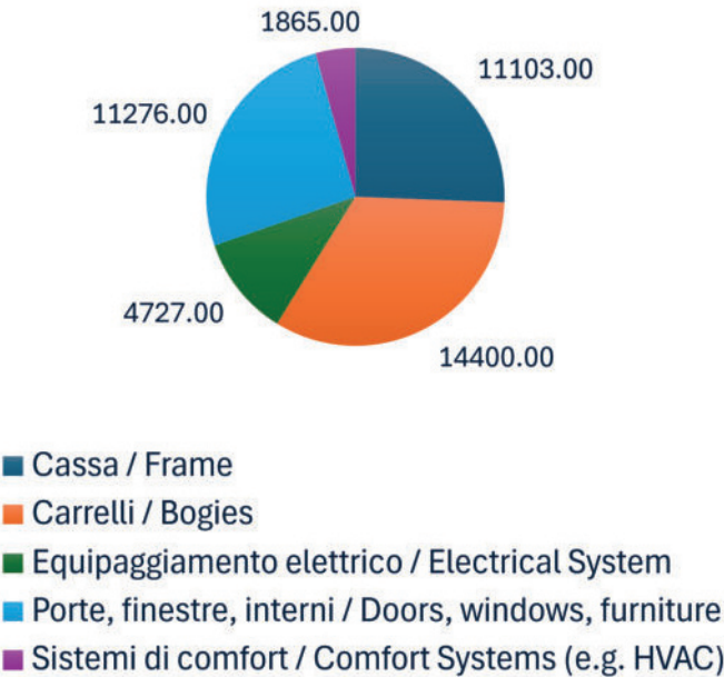
Figura 4 - Scomposizione della massa della carrozza in sottosistemi. Figure 4 - Breakdown of the coach mass into subsystems.
