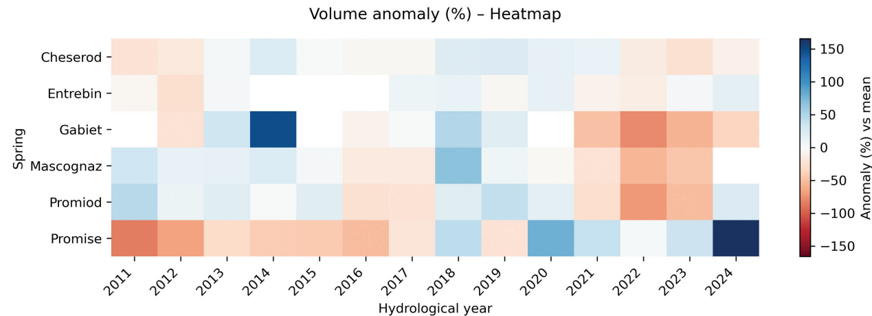
Fig. 5 - Heatmap of annual discharge anomalies (% vs. mean) for monitored springs (2011–2024). Fig. 5 - Mappa delle anomalie annuali di portata (% rispetto alla media) delle sorgenti monitorate (2011–2024).
