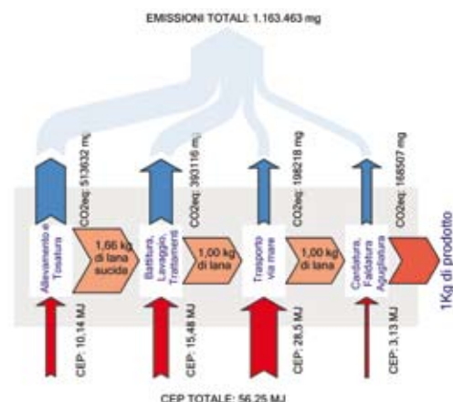
02 | Filiera di produzione di un isolante termo-acustico in lana di pecora proveniente dalla Nuova Zelanda
