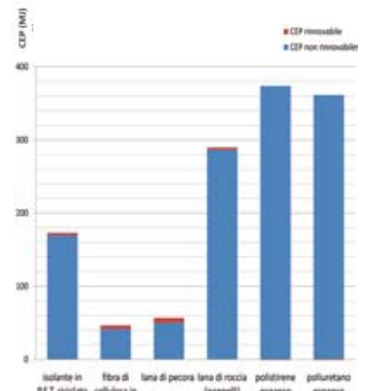
01 | L'istogramma confronta il Contenuto di Energia Primaria concernente l'isolamento termico di un involucro edilizio opaco. I dati si riferiscono all'energia necessaria per ottenere una trasmittanza termica di 0,24 W/m 2 K in una parete esterna verticale
