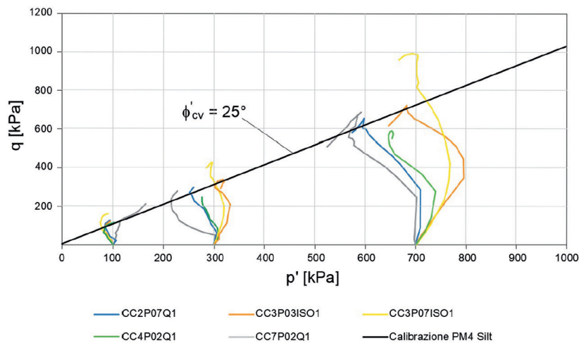
Figura 10. Risultati delle prove TX-CIU su campioni prelevati nello strato LA e proiezione della retta CSL nel piano q-p'.
