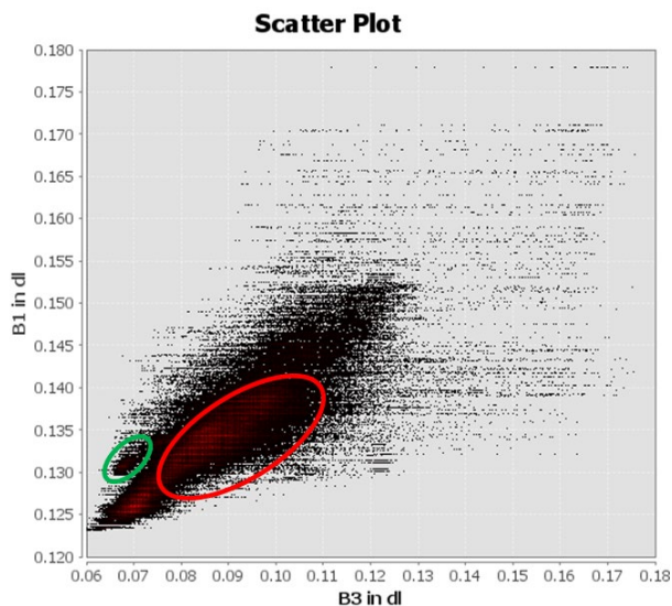
FIGURA 5. Scatter plot delle due bande B1 (coastal blu) e B3 (Green) dell'immagine di luglio 2022. Con le ellissi colorate si sono evidenziate le zone sul grafico corrispondenti a diverse zone geografiche, caratterizzate rispettivamente da valori più alti di B1 e meno alti di B3 (ellissi verde) e da valori meno alti di B1 e più alti di B3 (ellissi rossa).
