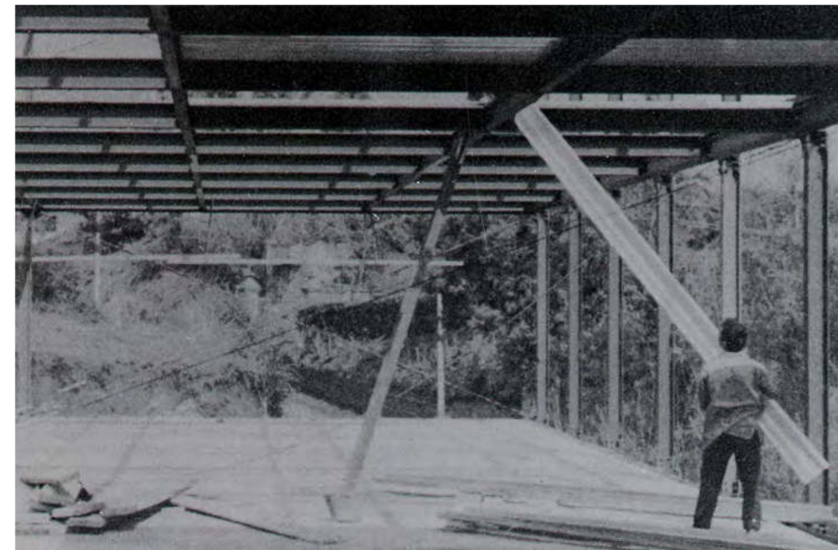
Foto del montaggio dei solai in acciaio nervato - dal cantiere dell'Istituto tecnico industriale prefabbricato di Velletri, con il sistema brevettato Tecnosider (scansioni A.C.S.). Photo of ribbed steel floor assembly - from the site of the prefabricated Industrial Technical Institute in Velletri, using the Tecnosider patented system (scans from C.S.A.).
