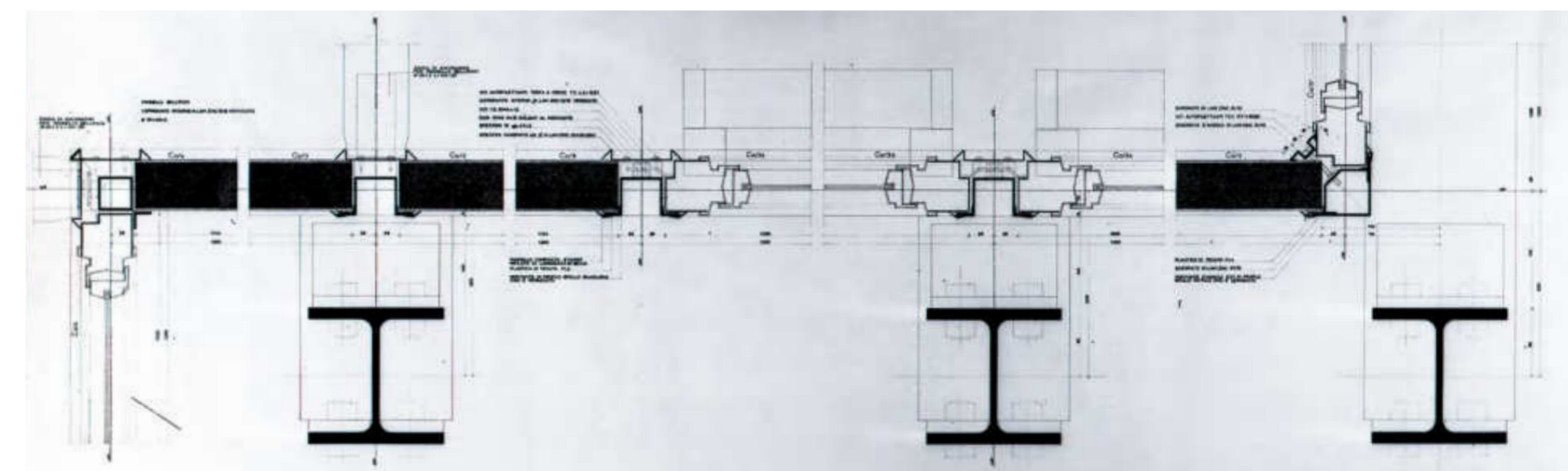
Planimetria dell'edificio in esame e dettaglio in pianta della facciata (scansioni A.C.S.).
