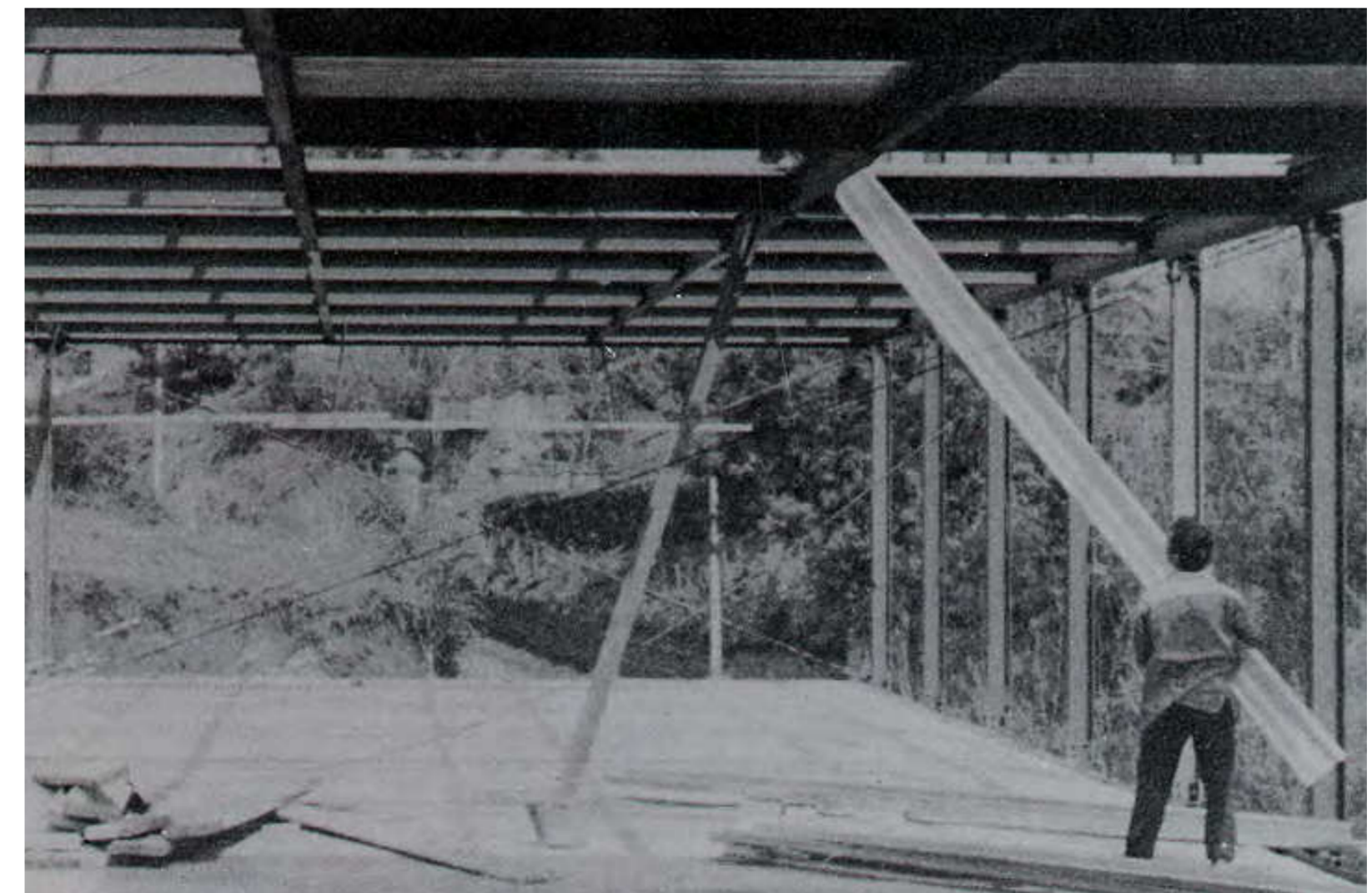
Foto del montaggio dei solai in acciaio nervato - dal cantiere dell'Istituto tecnico industriale prefabbricato di Velletri, con il sistema brevettato Tecnosider (scansioni A.C.S.).
