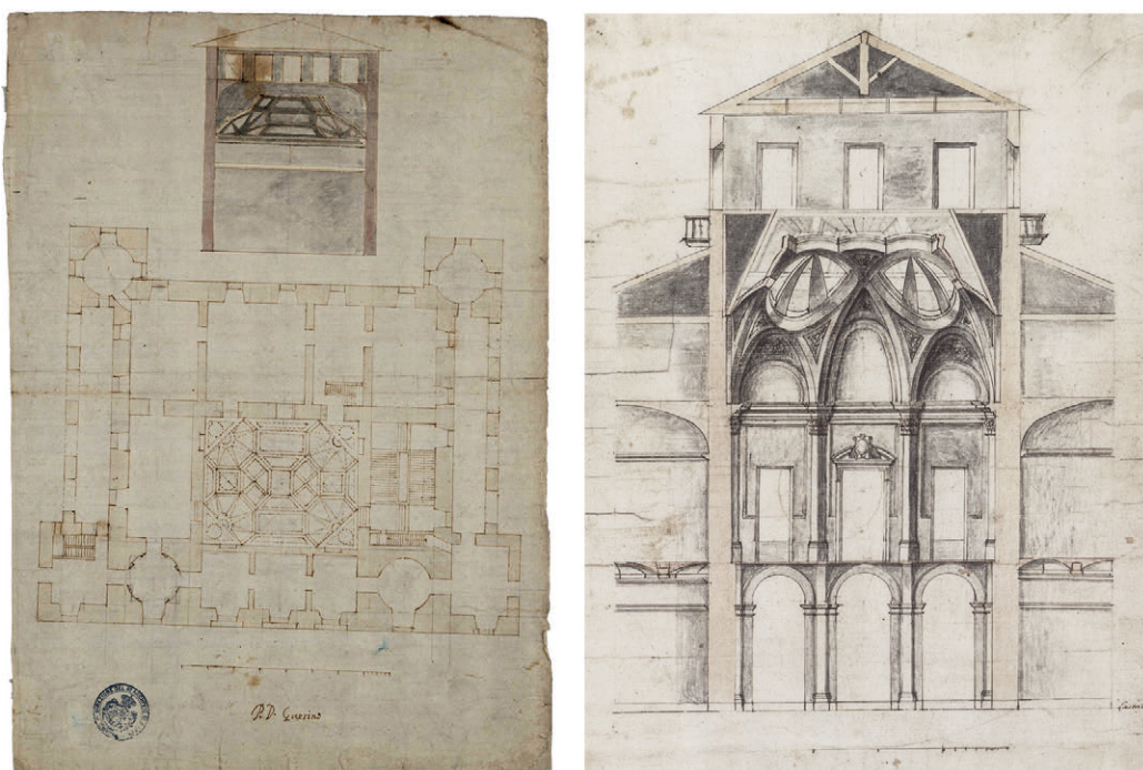
Fig. 6. A sinistra: studio per il salone di Palazzo Madama, c. 1675-1677. ASTR, Az. Sav.-Car., Palazzo Madama, maz. 16, fog. 1; a destra: studio per il salone del Castello di Racconigi, c. 1677. ASTR, Az. Sav.-Car., Castello Racconigi, maz. 73, fog. 1 (destra).
