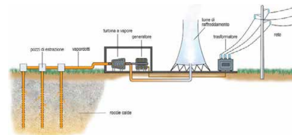
Schema di funzionamento di una centrale geotermica da https://educazionetecnicaonline.com
