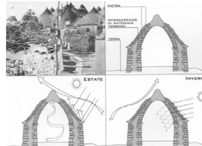
Foto e schema di funzionamento di un trullo da http://www.studioarchitetturaabp.it
