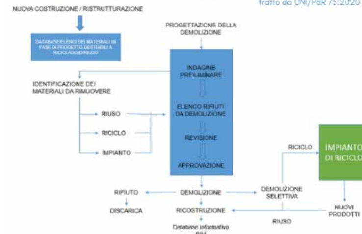
Schema processo demolizione selettiva – tratto da UNI PdR 75:2020
