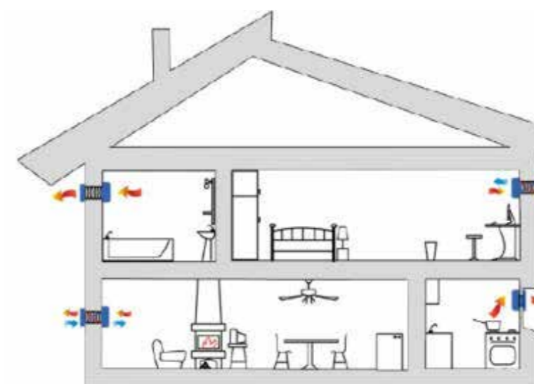
Schema impianto VMC decentralizzato da https://www.archimedegroup.eu
