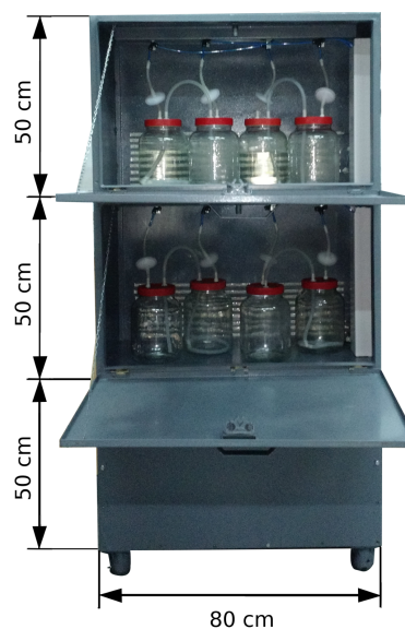
Fig. 2. Sistema de Inmersión Temporal desarrollado.
