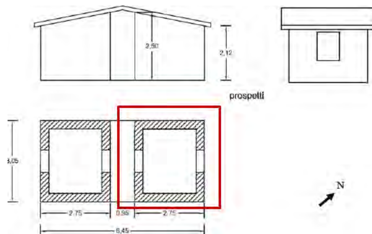
Figura 2. Geometria degli edifici test utilizzati nello studio.
