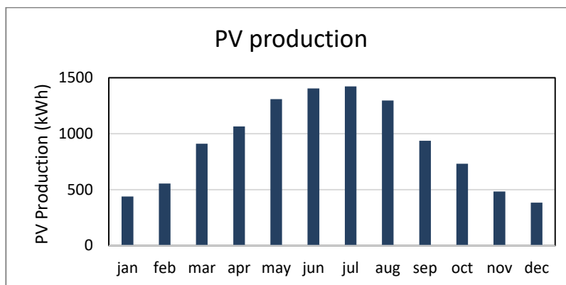
Figura 10. Produzione energetica mensile del generatore fotovoltaico.
