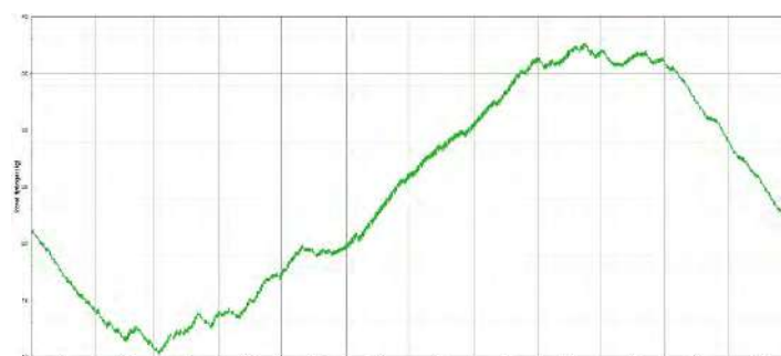
Figura 13. Massa di idrogeno stoccato nei vari mesi dell'anno.
