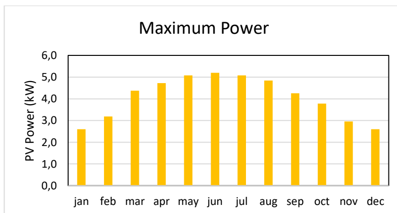
Figura 9. Potenza massima prodotta dall'impianto fotovoltaico.
