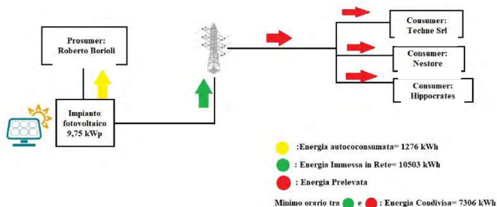
Figura 6. Analisi Energetica
