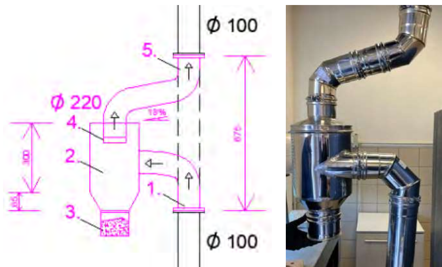
Figura 4. Ciclone Passivo – Vista Frontale.
