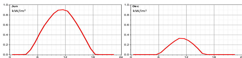
Figura 7. Intensità della radiazione solare oraria giornaliera media a Giugno e Dicembre.
