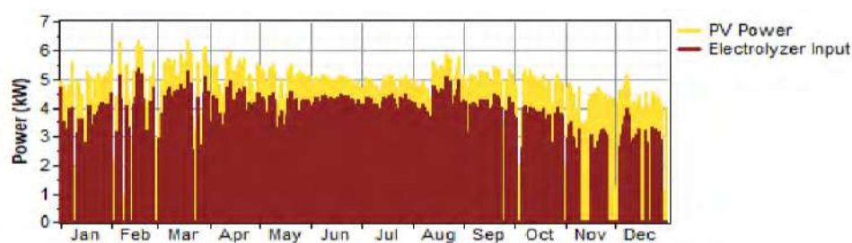
Figura 11. Potenza fotovoltaica oraria ed aliquota inviata all'elettrolizzatore.
