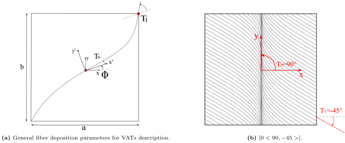
Fig. 1. Variable Angle Tow (VAT) representation.
