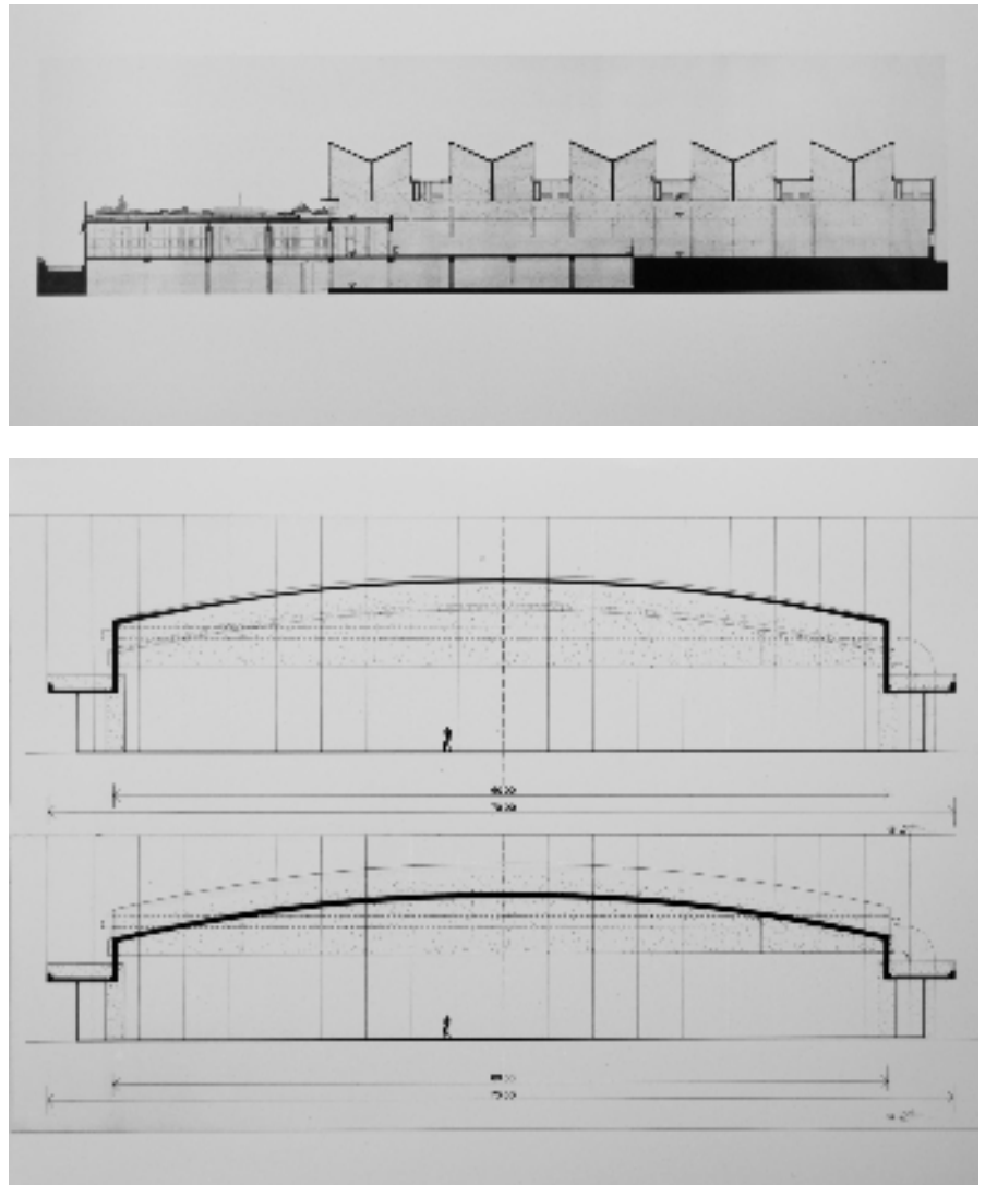
Figg. 12 Complesso Gandolfi-OM, San Lazzaro di Savena (Bologna), 1962–65. Sezione trasversale e longitudinale.
