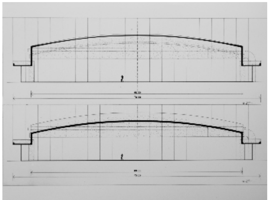
Fig. 12 Complesso Gandolfi-OM, San Lazzaro di Savena (Bologna), 1962–65. Sezione trasversale e longitudinale.
