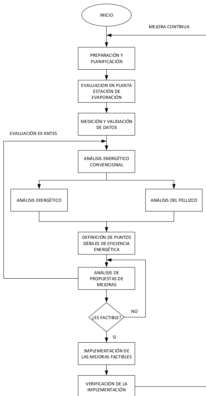
Fig. 2- Diagrama heurístico con la metodología para la evaluación de la eficiencia energética de la estación de evaporación de ingenios azucareros
