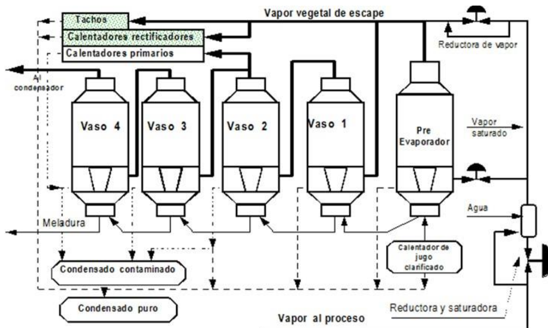
Fig. 1- Esquema típico de uso del vapor en una estación de evaporación de ingenios azucareros (11)
