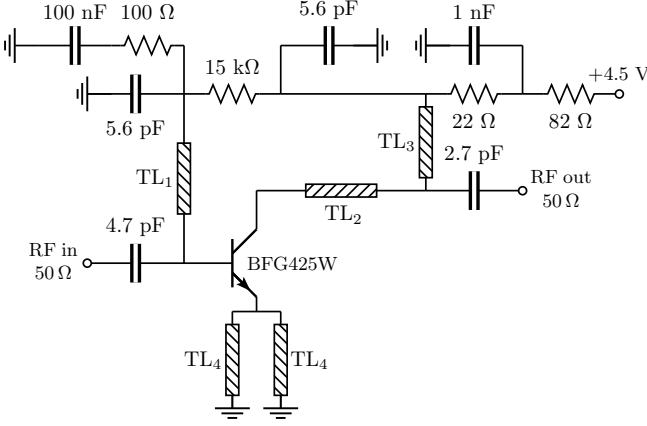
Fig. 1. 2-GHz BJT LNA.
