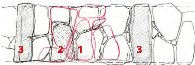
Figura 21 - Pianta
