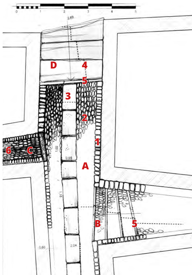
Figura 1 Pavimentazione lapidea a secco in villaggio rurale montano ossolano. Pianta, disegno originale in scala 1:50.
