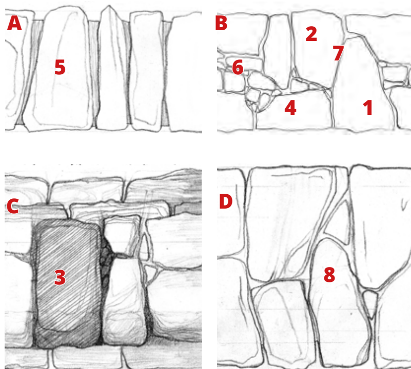
Figura 27 Sezioni orizzontali
