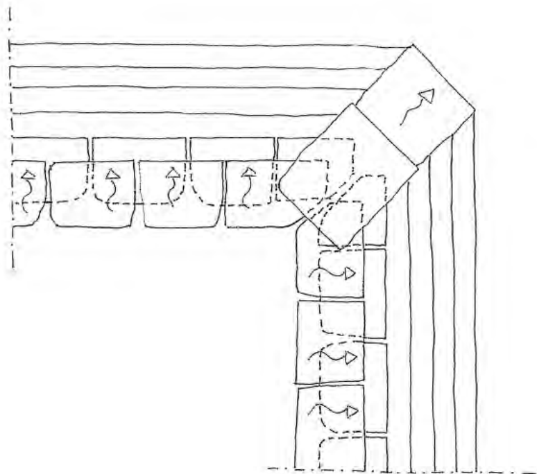
Figura 58 Espluvio angolare con pioda diagonale. 1 - Elemento di maggiore profondità rispetto alle altre piode del manto; 2 - Elemento idealmente concavo.
