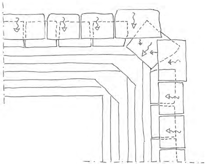
Figura 57 Impuvio angolare con pioda diagonale 1 - Elemento di maggiore profondità rispetto alle altre piode del manto; 2 - Elemento idealmente concavo.
