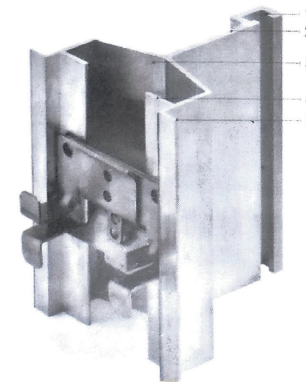
Porzione di un montante metallico con apposite “manine” per il fissaggio delle tavole da Campioli A., Lavagna M. (2013), Tecniche e architettura , Città Studi
