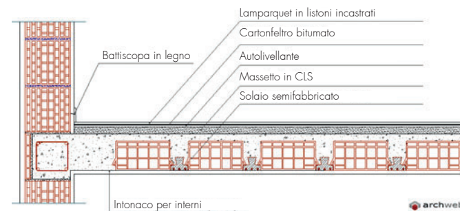
Esempio di solaio in laterocemento da http://www.maxb.it/immagine-particolare-rete-metallica-dwg-canniccio-bambu-26047/
