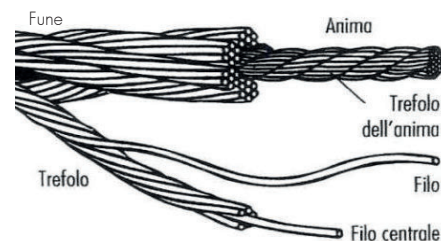
Esplosio di una fune di acciaio per tensostrutture da https://www.regione.vda.it/alegato.aspx?pk=44722
