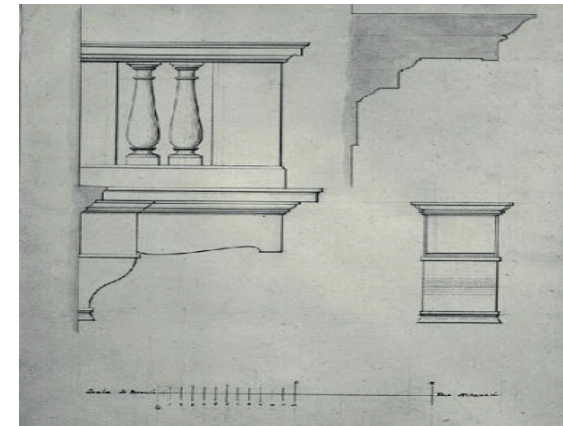
Prospetto laterale del balcone con ingrandimento sui modiglioni da http://www.lombardiabeniculturali.it/img_db/bcoa/4y010/22/1/21404_127750010
