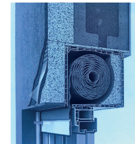
Spaccato assonometrico di un architrave costituito da due pannelli isolanti a L da Campioli A., Lavagna M. (2013), Tecniche e architettura , Città studi
