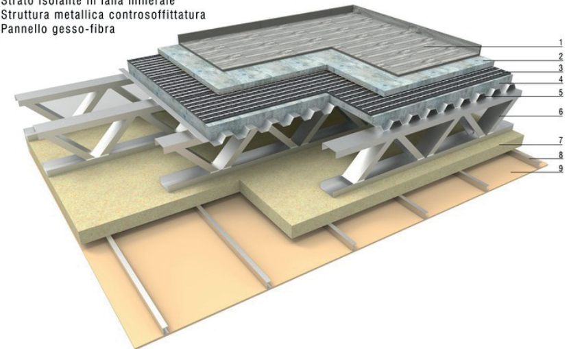
Solaio in lamiera grecata da https://www.ideabuilding.it/totale-assenza-di-muffe-e-umidita/
