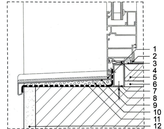
Componenti del davanzale da CAMPIOLI A., LAVAGNA M. (2013), Tecniche e architettura , Città Studi
