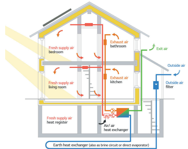
Impianto di ventilazione controllata da https://www.lgbusiness.it/magazine/climatizzazione/passive-house-la-casa-che-crea-nuovi-standard-di-efficienza/
