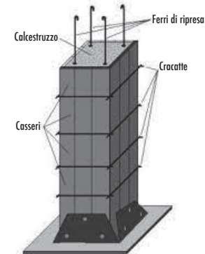
Disegno di un pilastro in calcestruzzo armato da https://www.google.com/url?sa=i&url=https%3A%2F%2Fwww.infub.com
