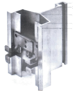
Porzione di un montante metallico con apposite “manine” per il fissaggio delle tavelle da Campioli A., Lavagna M. (2013), Tecniche e architettura , Città Studi
