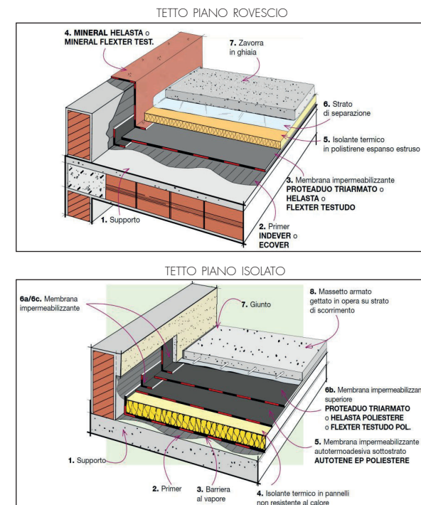
Tipologie di tetto piano da https://www.indexspa.it/IT/stratigrafia.asp?ids=29
