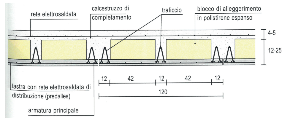
Solaio misto semiprefabbricato a lastre Predalles con blocchi alleggeriti in polistirolo espanso da Arbiziani E. (2015), Tecnica e tecnologia dei sistemi edilizi , Maggioli Editori
