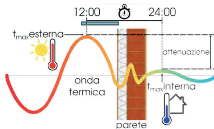
Sfasamento termico da http://www.unife.it/architettura/lm.architettura/insegnamenti/laboratorio-di-costruzione-dellarchitettura-i
