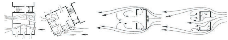
Dimostrazione di orientamento dell'edificio per sfruttare il vento da https://www.architetturaecosostenibile.it/architettura/criteri-progettuali/ventilazione-naturale-come-si-fa-ottenere-le-finestre
