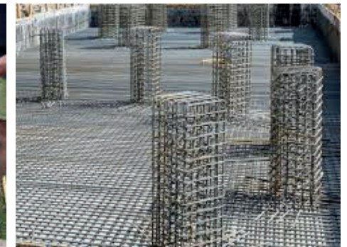
Armatura ancora a vista di pilastri e soletta da https://www.google.com/url?sa=i&url=https%3A%2F%2Fwww.ingegneri
