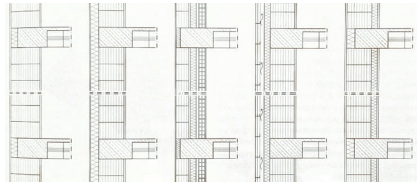
Tipi di chiusure da CAMPIOLI A., LAVAGNA M. (2013), Tecniche e architettura , Città Studi
