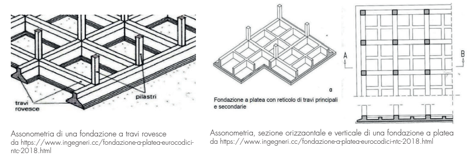
Fondazione continua a cordolo e a trave rovescia rielaborazione da Campioli A., Lavagna M. (2013), Tecniche e architettura , Città Studi Sezione di trave a cordolo da Arbizzani E. (2015), Tecnica e tecnologia dei sistemi edilizi. Progetto e costruzione , Maggioli Editore
