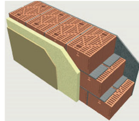
Muratura portante in laterizio da http://www.poraton.it/soluzioni-costruttive/murature-portanti-in-laterizio.aspx
