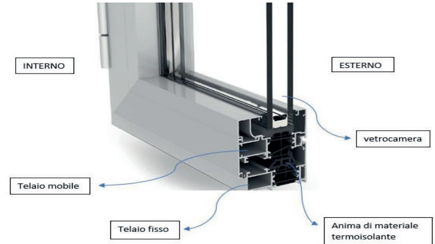
Telaio a taglio termico rielaborazione da https://www.aluroma.com/infissi-in-alluminio-a-taglio-termico-cosa-sono-e-perche-scegliarli/
