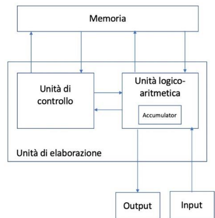
Fig. 3 – Schema dell'Architettura di von Neumann
