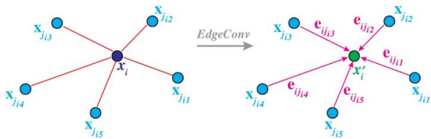
Figura 3. Modulo EdgeConv . L'output di EdgeConv viene calcolato aggregando le features del bordo associate a tutti i bordi provenienti da ciascun vertice connesso.
