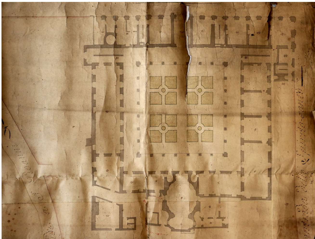
fig. 4 – Planimetria del piano terreno del complesso del Seminario, prima degli interventi di stravolgimento commissionati a Carlo Ceroni (ASMT, Carte e Disegni , 8, «Maison du Seminaire de Turin n.1 Seminario»).
