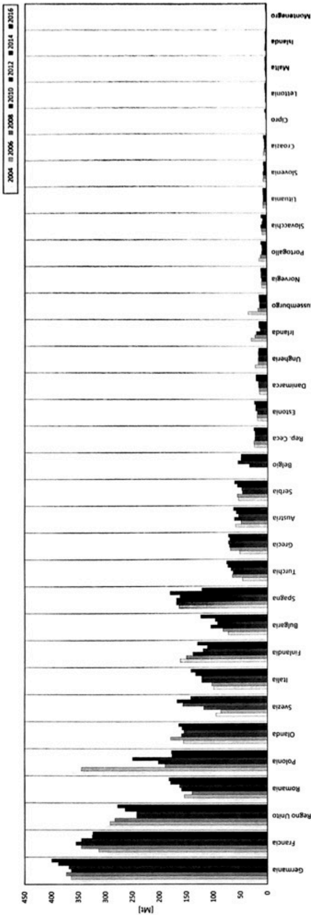
Fig. 1. Produzione di rifiuti solidi (pericolosi e non pericolosi) in EU-28 i tra il 2004 e il 2016 (Eurostat, 2020). Production of solid waste (hazardous and not hazardous) in EU-28 between 2004 and 2016 (Eurostat, 2020).
