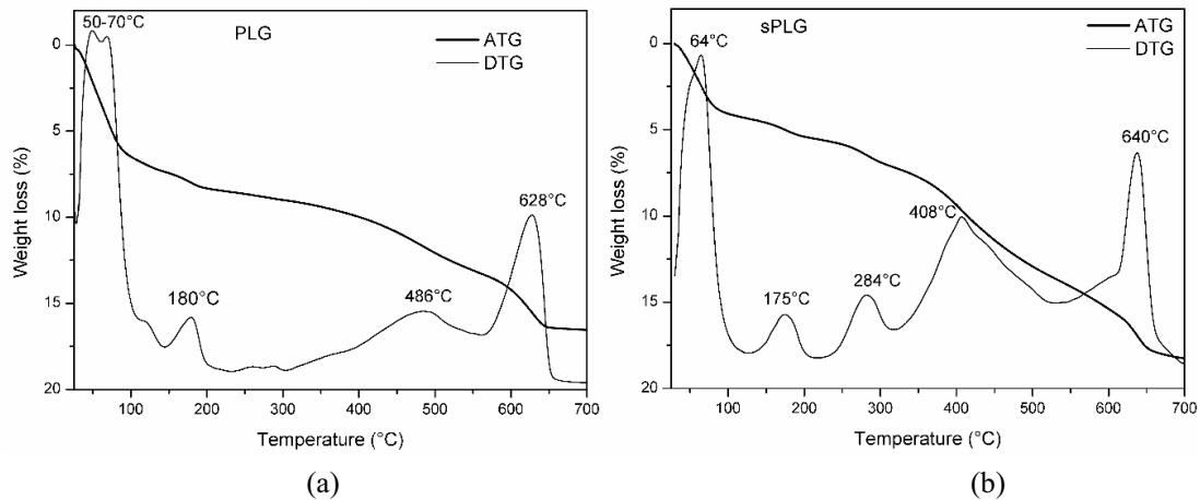
Figure 4: Thermogravimetric curves of (a) PLG and (b) sPLG nanofillers
