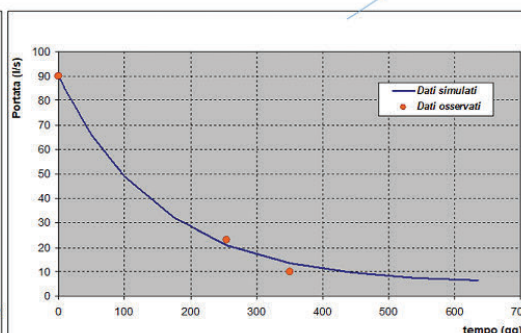
Fig. 3 - Analisi delle venute d'acqua osservate in opere sotterranee già realizzate.
