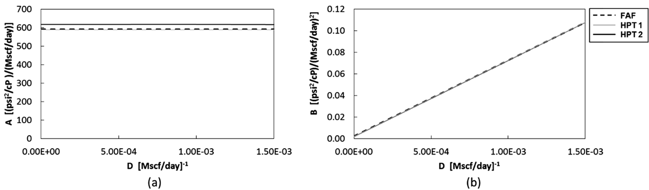
Fig. 12. Comparison of HPT configurations (solid lines) and FAF test (dotted line) in terms of estimated (a) non-turbulent and (b) turbulent component coefficients. Confronto tra le diverse configurazioni di HPT considerate (linee continue) ed il FAF test (linea tratteggiata) in termini di stima dei coefficienti di componente (a) non-turbolenta e (b) turbolenta.
