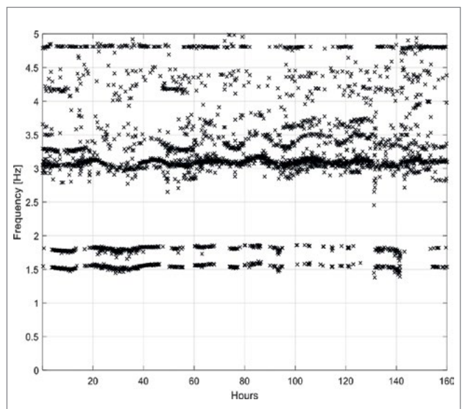
Figura 22 Frequenze modali estratte durante una settimana di monitoraggio.
