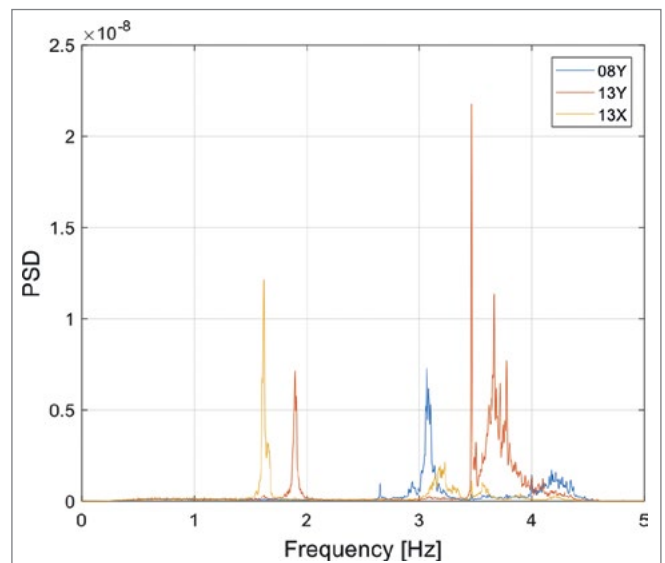
Figura 17. Contenuto in frequenza registrazione del 02/06/2017, ore 18-19.
