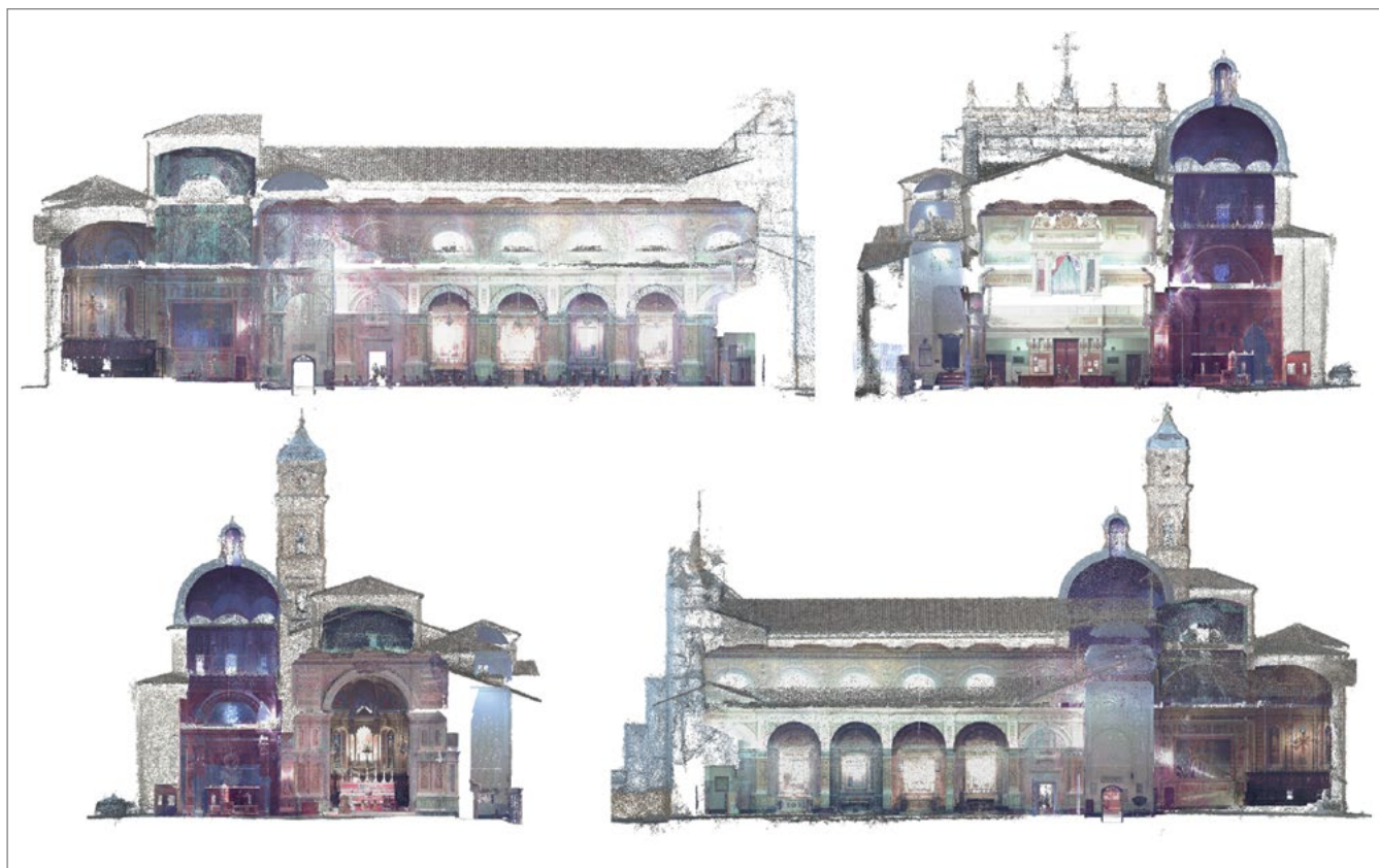
Figura 13. Sezioni longitudinali e trasversali, derivate dalle nuvole UAV e TLS integrate, utilizzando piani sezione tipici della rappresentazione architettonica.
