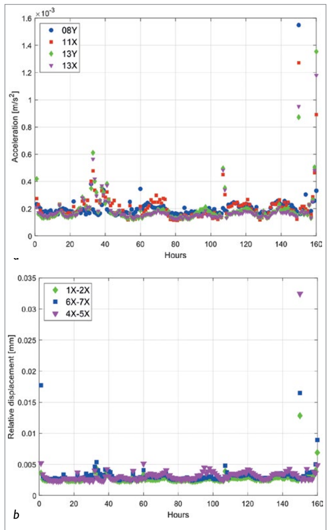
Figura 21. (a) RMS delle accelerazioni acquisite sulla struttura; (b) RMS degli spostamenti relativi tra facciata e navata e tra facciata e abside.
