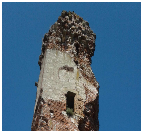
Fig. 4. Battifollo (CN): i ruderi della torre con i chiari segni di degrado e dissesto delle strutture murarie.
