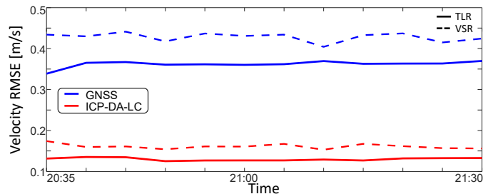
b) Velocity
