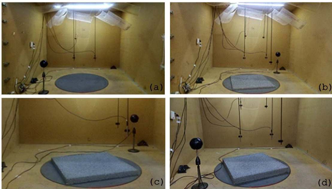
Figura 3 – Camera riverberante in scala 1:5 senza il campione (a) e con il campione A (b), con il campione B (c) e con il campione C (d) (Dip. di Energia, Politecnico di Torino) – 1:5 scaled reverberation room without the sample (a) and with the measured sample A (b), Sample B (c) Sample C (d) (Dep. of Energy, Politecnico di Torino).
