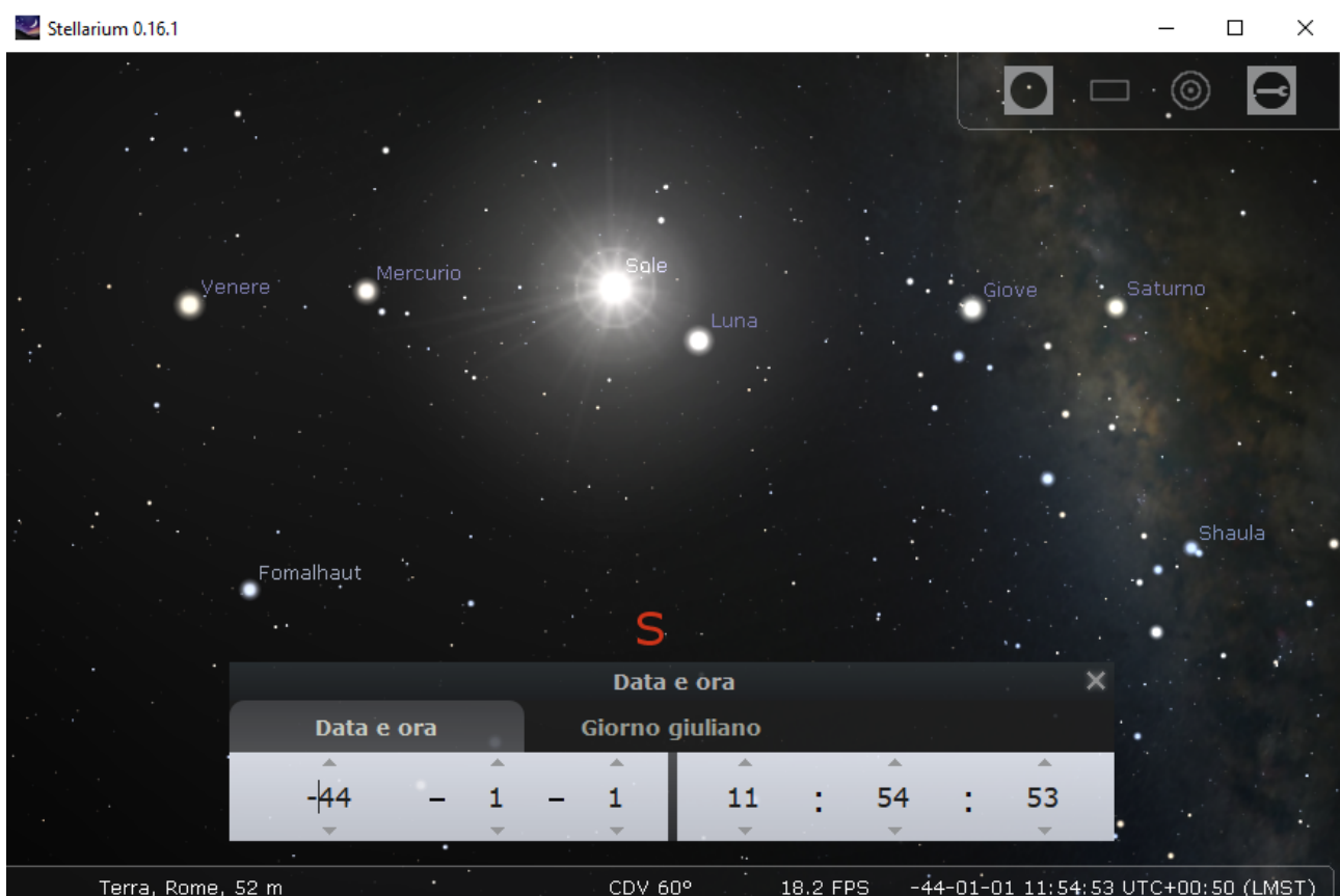
Figura 1: Il cielo in Stellarium il primo Gennaio del 45 a.C. . Interessante sequenza di corpi celesti: Venere, Mercurio, Sole, Luna, Giove e Saturno. Il giorno 2 Gennaio la sequenza è Venere, Mercurio, Luna, Sole, Giove, Saturno.
