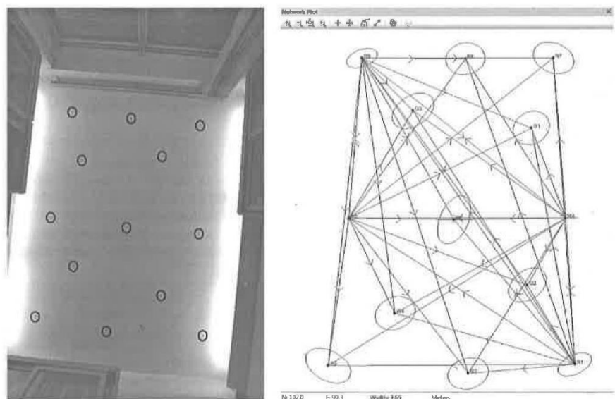
Fig. 2. Reference system – circles evidence the markers (left), Least Square network adjustment with error ellipses (right). Sistema di riferimento – i cerchi evidenziano i markers (sinistra), compensazione del sistema di riferimento con metodo ai Minimi Quadrati con ellissi d'errore (destra).
