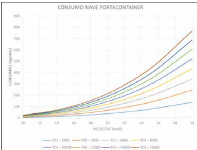
FIG. 12 ESEMPIO DI ANDAMENTO DEI CONSUMI, ESPRESI IN TBUNKER/GIORNO, DI UNA NAVE PORTACONTAINER AL VARIARE DELLA VELOCITÀ E DEL PESO (WWW.MATEMATICAMENTE.IT)
