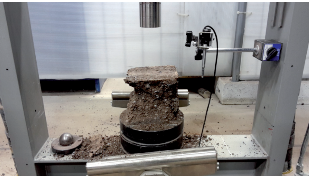
FIG. 2 Prova di compressione Unconfined compressive strenght test
