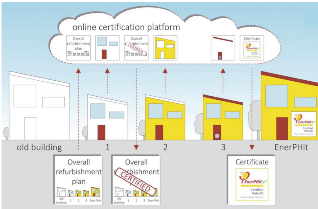
FIG. 1 Schematizzazione del processo di certificazione step-by-step EuroPHit per progetti di retrofit energetico Diagram of the EuroPHit step-by-step certification process for energy retrofit projects
