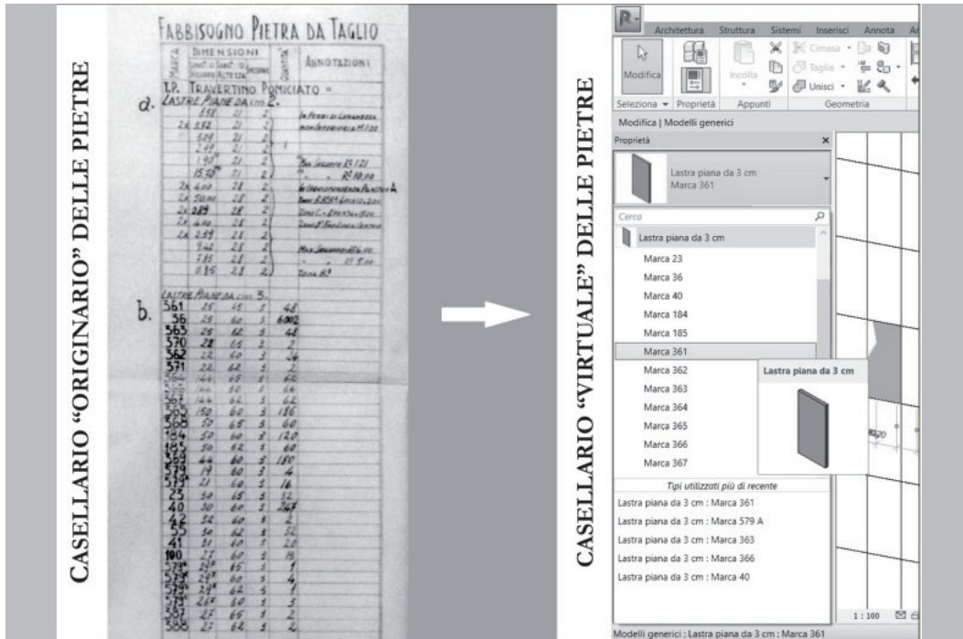
FIG. 2 Dal Casellario "originario" delle pietre a quello "virtuale": gli oggetti HBIM delle lastre del rivestimento lapideo From the "original" Abacus of stones to the "virtual" one: the HBIM objects of stone facing sheets
