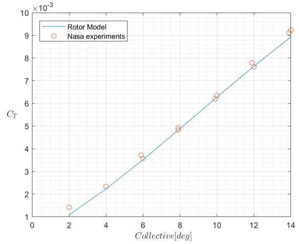
Fig. 15 UH-60 C_T - \theta trend in Hover
