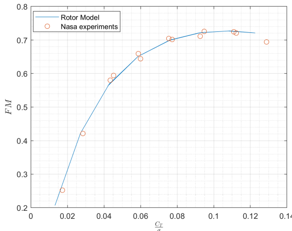
Fig. 16 UH-60 FM - C_T trend in Hover
