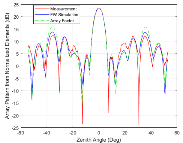
Fig. 4. preAAVS1 array (beam) patterns at 350 MHz.
