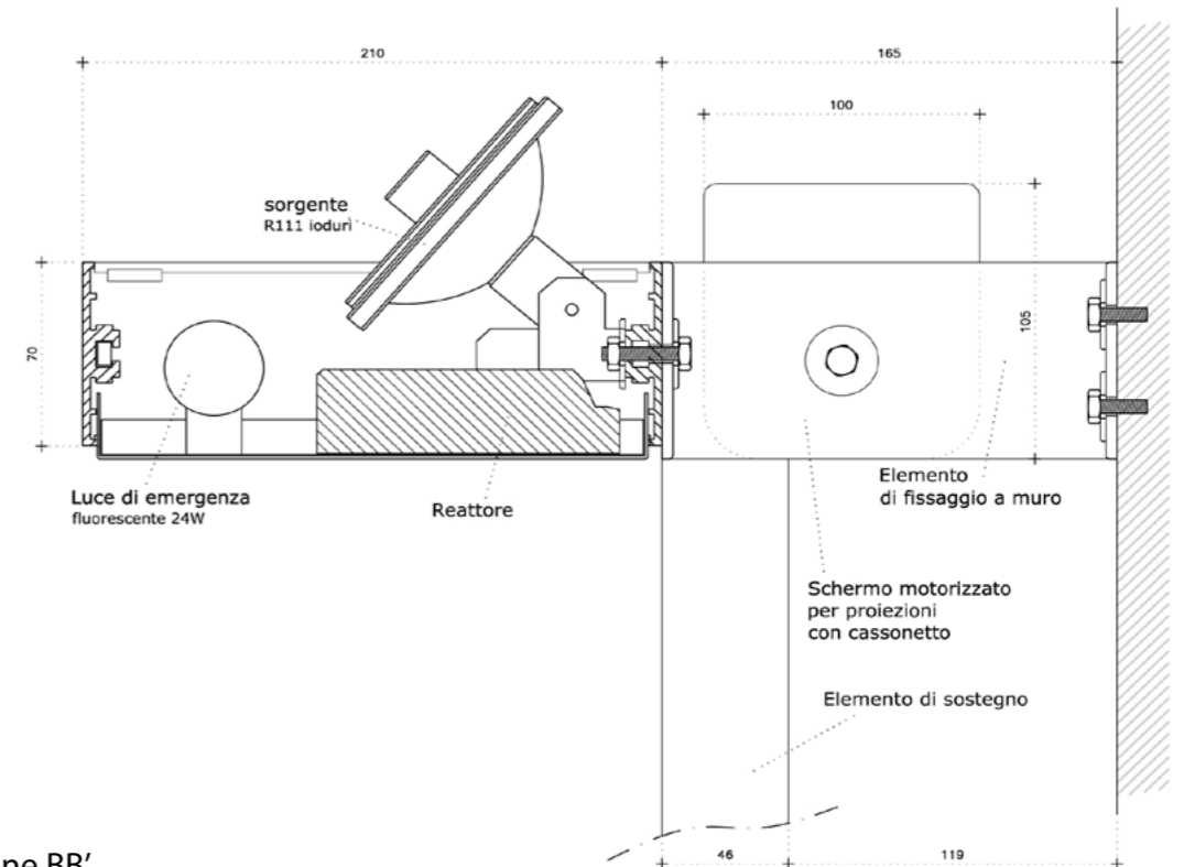
sezione BB'
