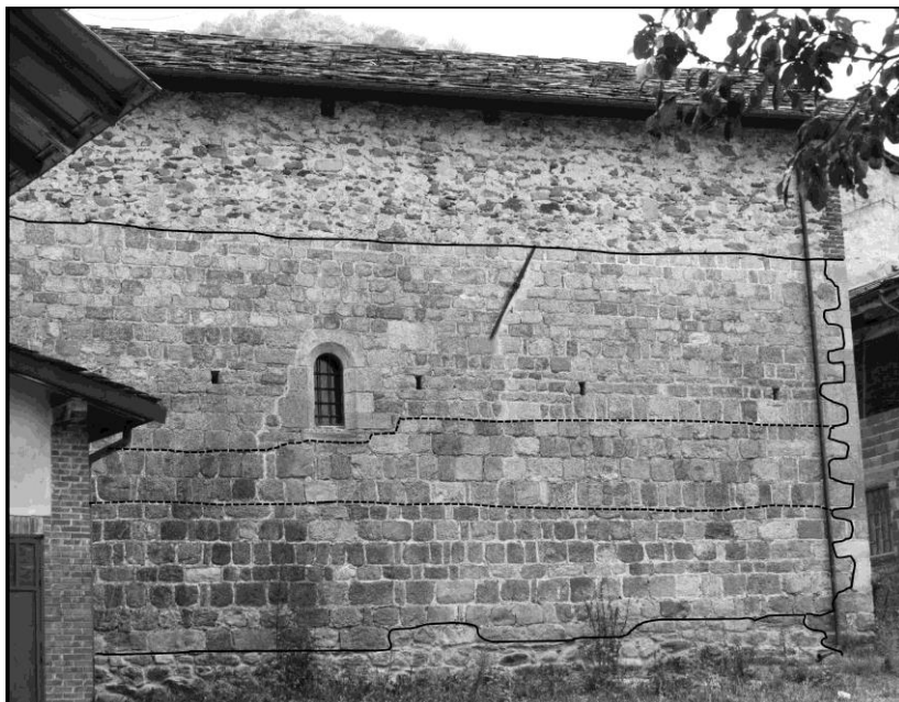
Fig. 2. Chiesa Pesio (Cuneo), correria della Certosa di Pesio. Prospetto laterale della chiesa con individuazione delle tessiture murarie. Le linee continue indicano una diversità nella costituzione dei filari, nelle dimensioni dei conci litici e nella loro apparecchiatura, corrispondenti a fasi di cantiere; le linee tratteggiate individuano modifiche meno rilevanti imputabili a scelte operate dalle maestranze per il posizionamento del materiale in rapporto alla disponibilità sul cantiere, non necessariamente corrispondenti a cronologie differenziate.
