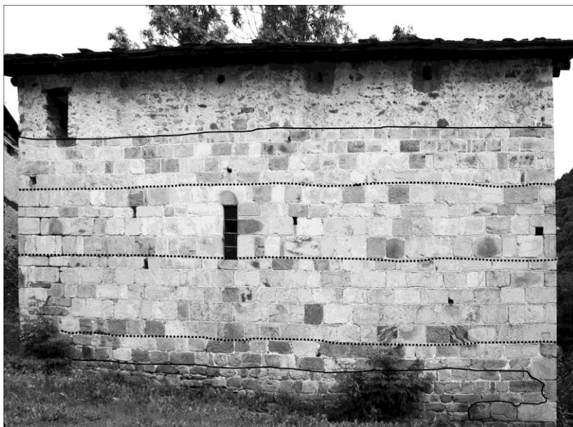
Fig. 4. Garessio (Cuneo), correria della Certosa di Casotto. Prospetto laterale della chiesa con l'identificazione delle fasi costruttive desunte dall'analisi delle tessiture murarie.
