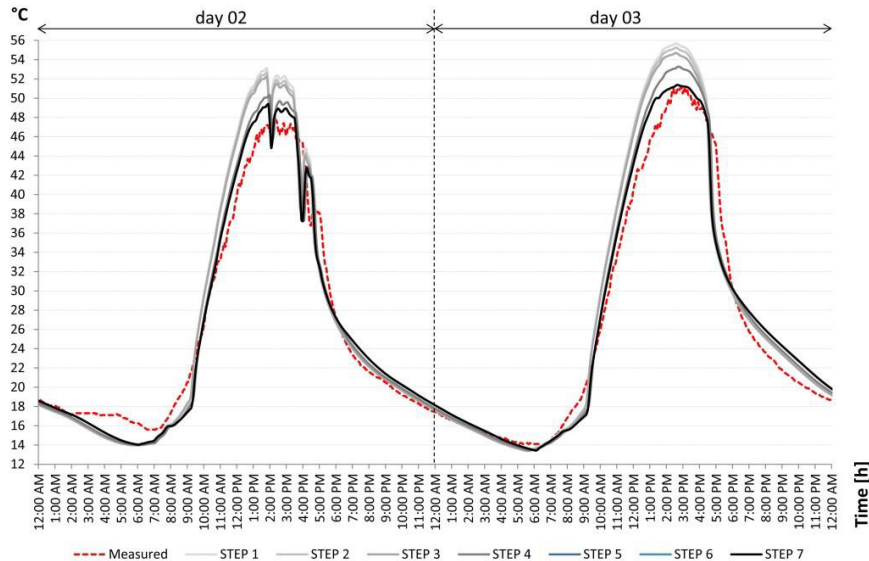
Fig. 4. T_{se} profile.
