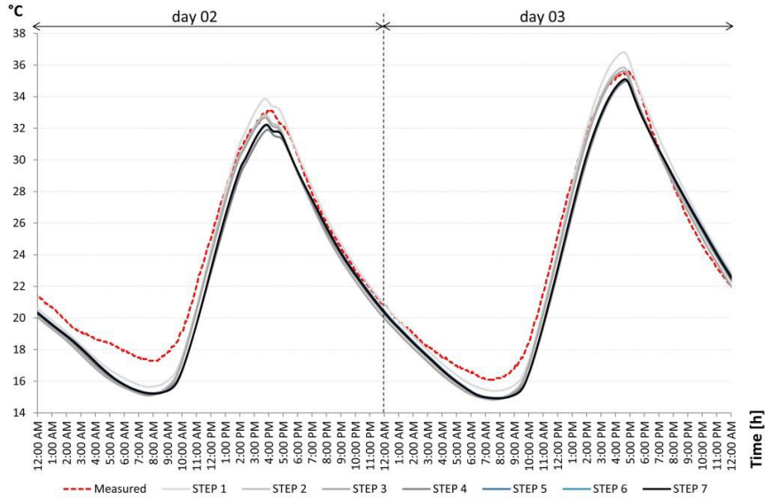
Fig. 5. T_{s2} profile.
