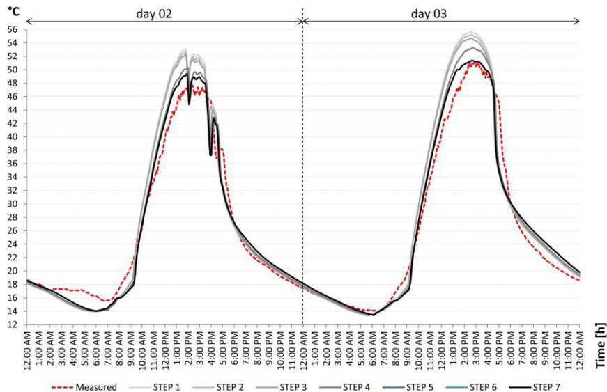
Fig. 4. T_{se} profile.
