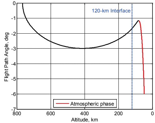
Fig. 6: FPA versus altitude.
