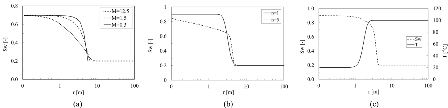
Figura 3: Effetto (a) del rapporto di mobilità ( M ) [10] e (b) dell'esponente ( n ) delle curve di permeabilità relativa sul fronte di spiazzamento nel caso di iniezione di acqua in un giacimento a olio; (c) confronto tra il fronte di saturazione del fluido spiazzante ( S_w ) e il corrispondente fronte termico ( T ) [11].
