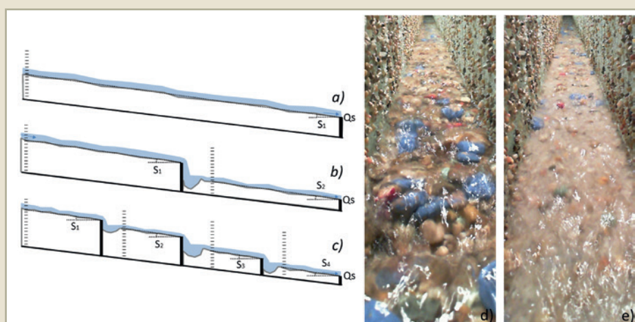
FIGURA 1 Schema dei diversi dispositivi: a) Ref Test; b) 1CD Test; c) 3CD Test – e stati estremi dell'alveo –; d) alveo pavimentato di sedimenti grossolani; e) letto ricoperto di sedimenti fini durante lo scorrimento in falde di fondo.
