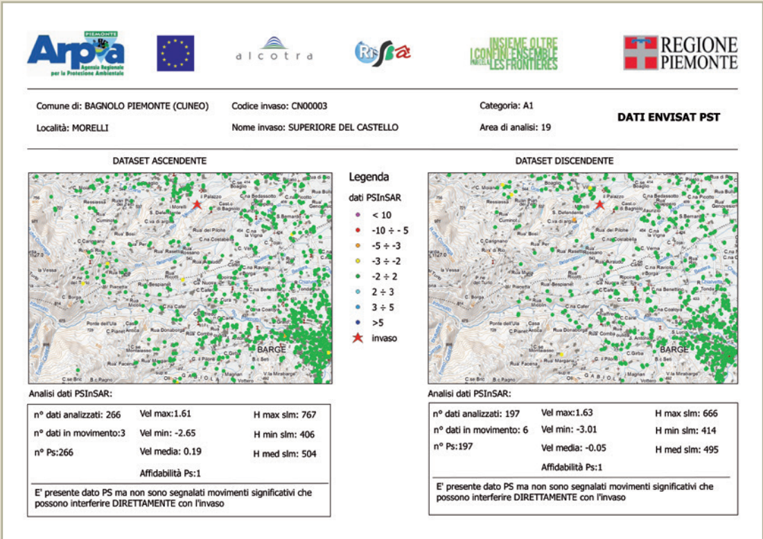
FIGURA 5 Layout per un invaso-tipo, copertura ENVISAT.
