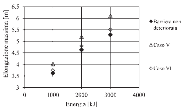
Fig. 8. Elongazione massima della barriera studiata per differenti livelli energetici di impatto e per i diversi casi di ammaloramento: casi V – VI rottura di un ancoraggio di monte.
