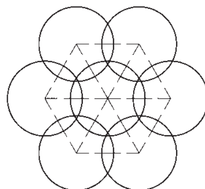
Fig. 3. Schema della modellazione della rete ad anelli con una rete equivalente esagonale.
