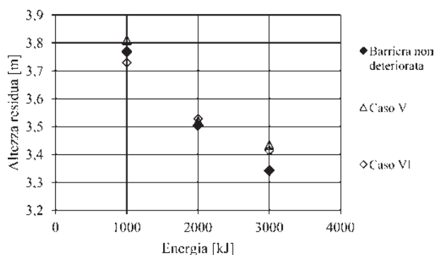
Fig. 10. Altezza residua della barriera studiata per differenti livelli energetici di impatto e per i diversi casi di ammaloramento: casi V – VI rottura di un ancoraggio di monte.
