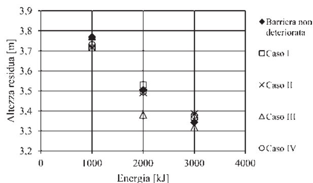
Fig. 9. Altezza residua della barriera studiata per differenti livelli energetici di impatto e per i diversi casi di ammaloramento: casi I – IV rottura di un controvento di monte.
