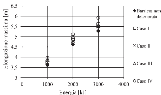
Fig. 7. Elongazione massima della barriera studiata per differenti livelli energetici di impatto e per i diversi casi di ammaloramento: casi I – IV rottura di un controvento di monte.
